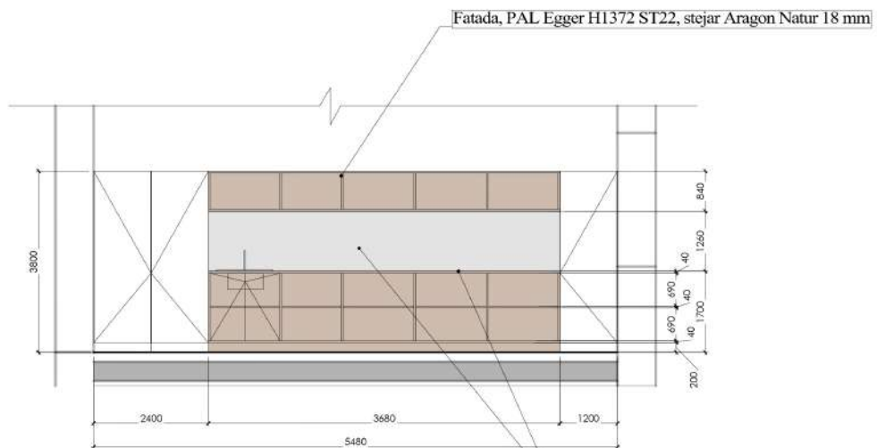
Vedere Frontala
