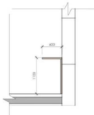
Sectiune A-A
