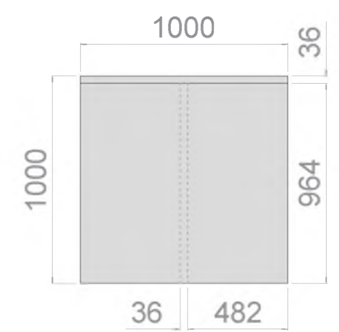
vedere laterala
