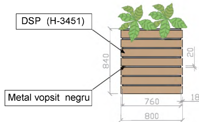
vedere frontala
