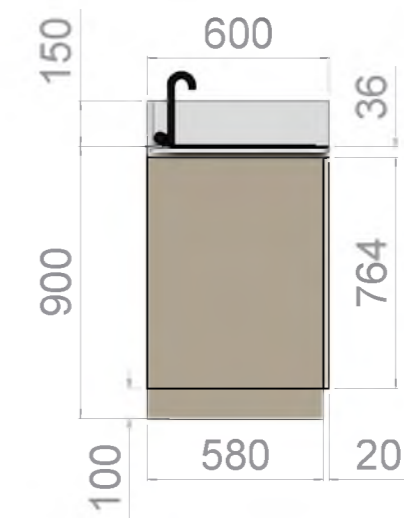
vedere laterala
