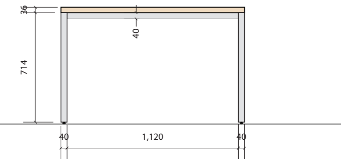
Vedere laterala
