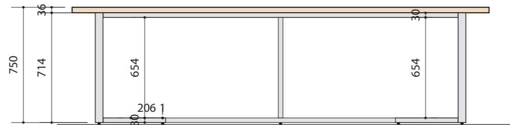
Vedere laterala
