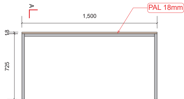
Vedere frontală
