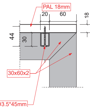
Detaliu 1, scara 1:25
