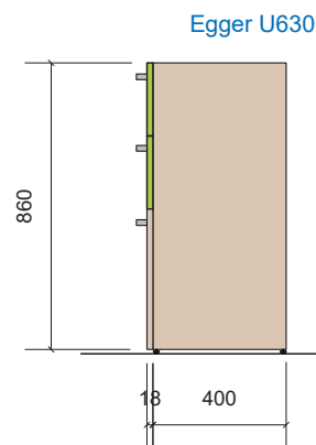
Vedere laterală
