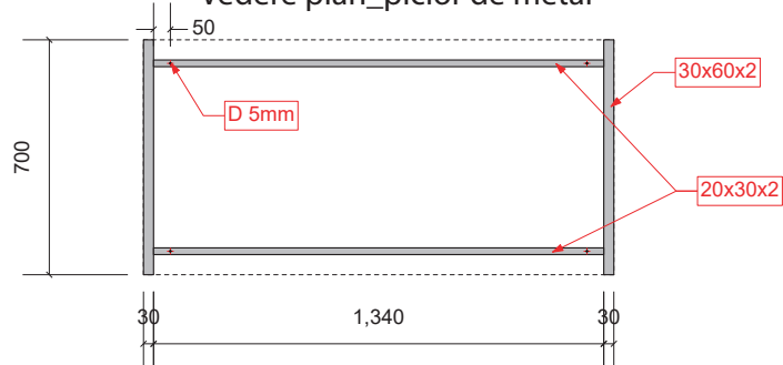
Vedere plan_picioar de metal
