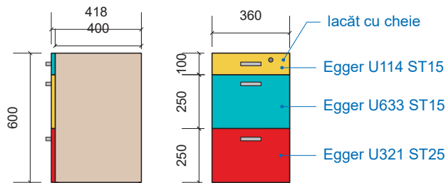
Dulap pentru masa_1_20 buc.
