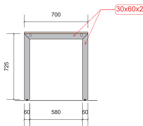
Vedere laterală
