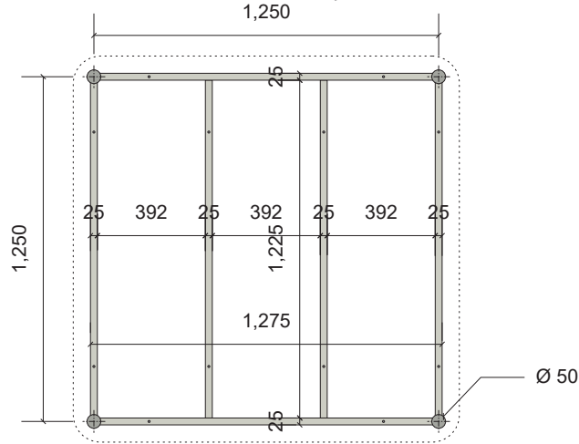
Vedere plan construcție metal
