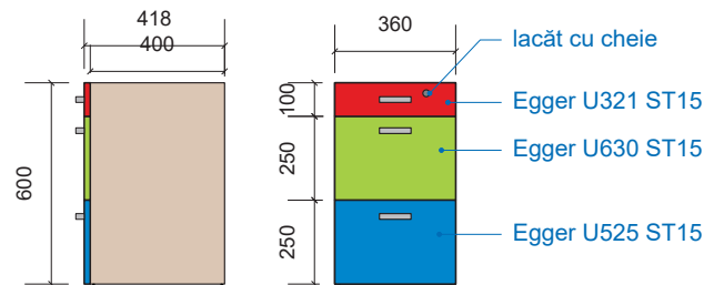
Dulap pentru masa_1_14 buc.
