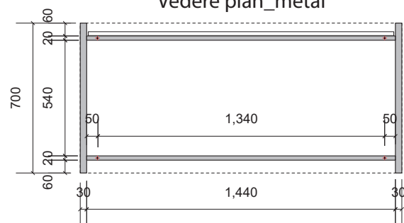
Vedere plan_metal
