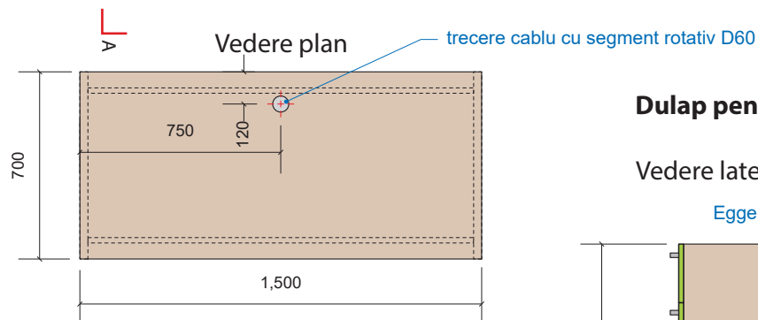
Vedere plan_metal
